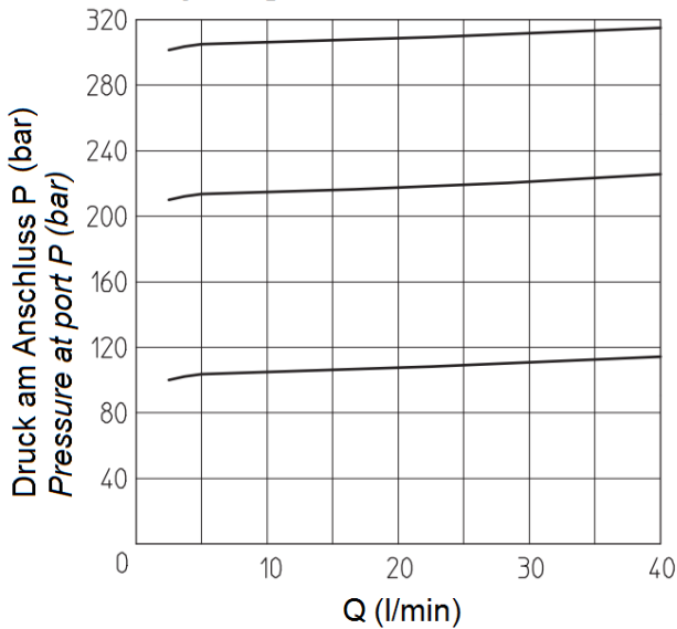
Q / p Kennlinie HK RZMO AE 030 Q / p diagram HK RZMO AE 030
