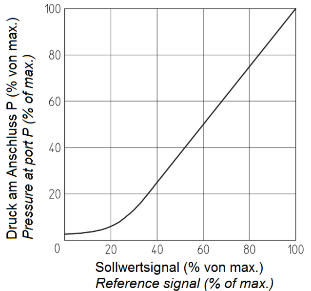
Regelkennlinie HK RZMO AE 030 Regulation diagram HK RZMO AE 030
